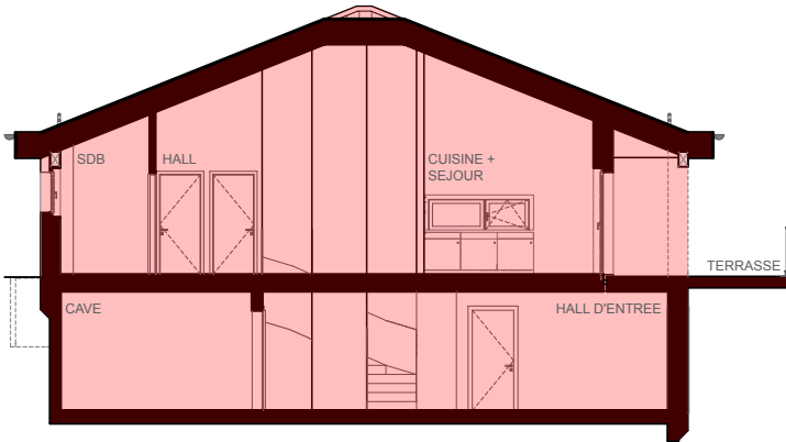
COUPE
